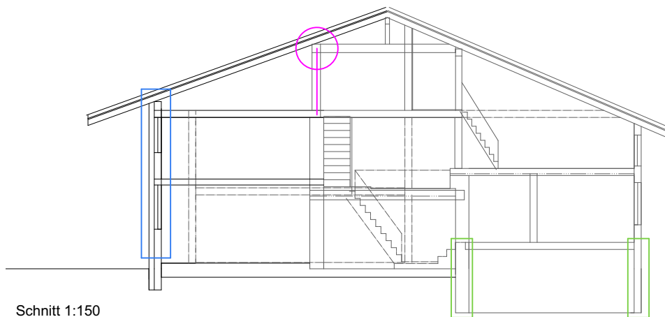
Schnitt 1:150
